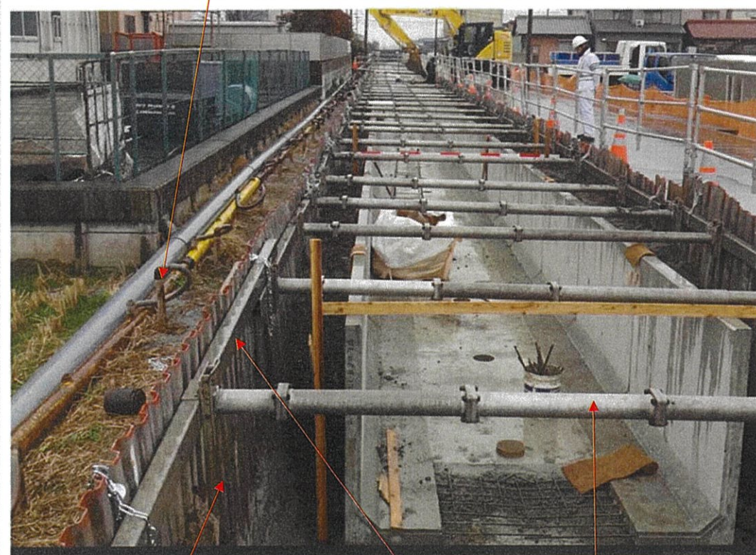
ウェルポイント工法
